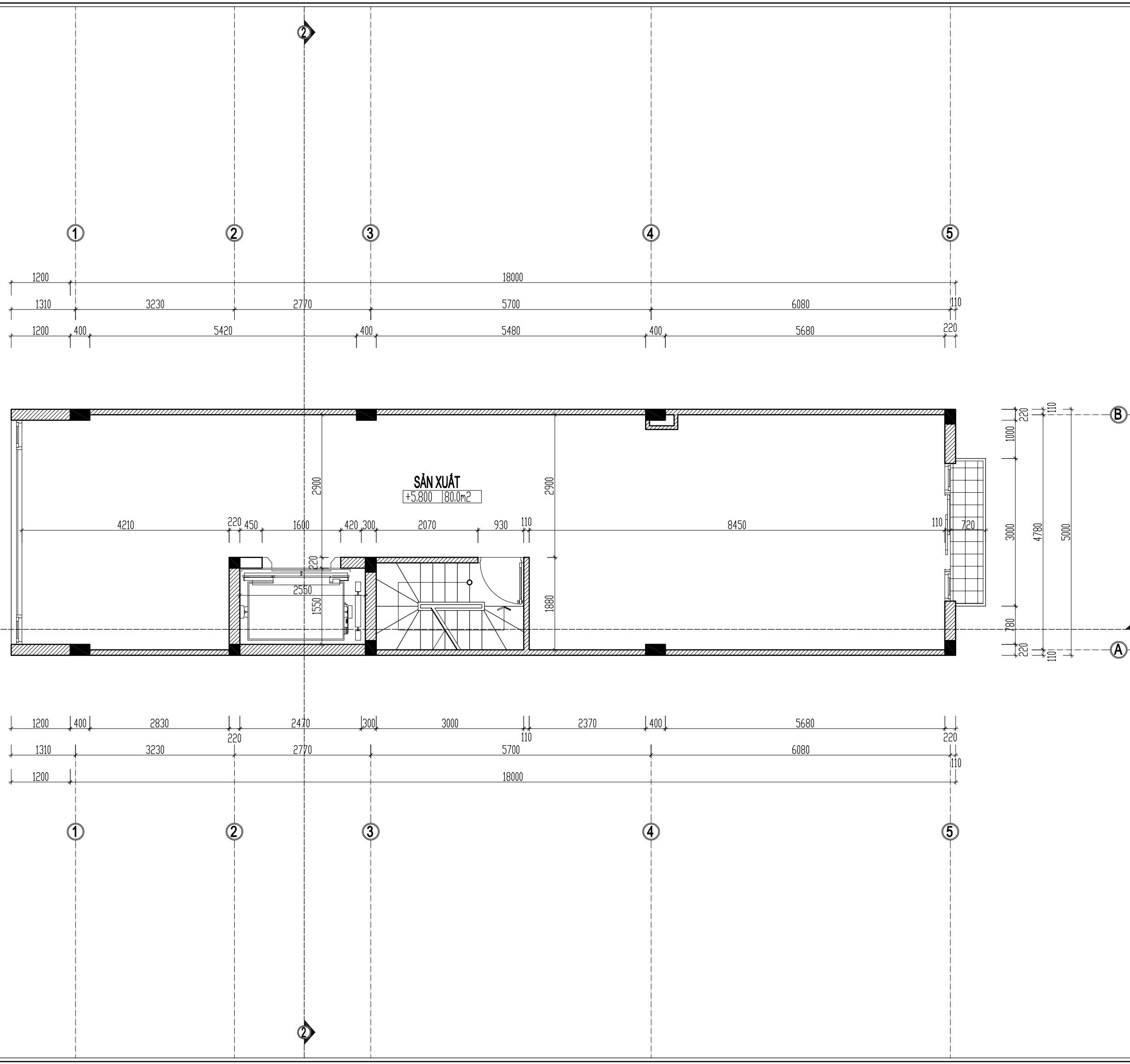
MẶT BẰNG TẦNG 2 +5.800 98.0m 2
